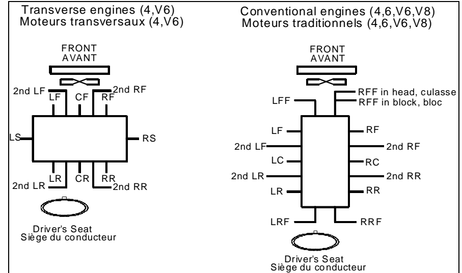
Location of Heater (from driver's seat) Position de la chaufferette (du siège du conducteur)
