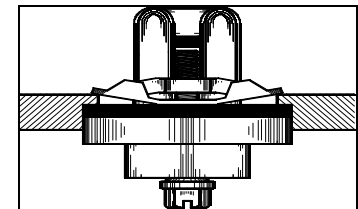
Figure 3 - Chauffe-bloc bien serré dans le bloc.
