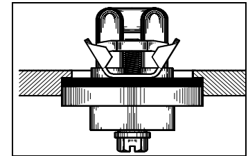
Figure 2 - Chauffe-bloc fermement placé contre le bloc.
