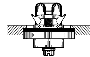
Figure 2 - Chauffe-bloc fermement placé contre le bloc.
